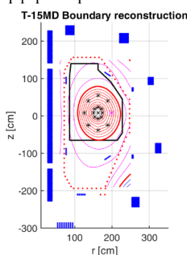
Рисунок 1 Пример восстановления равновесия в плазме Т15-МД, #845 (350 мс)
