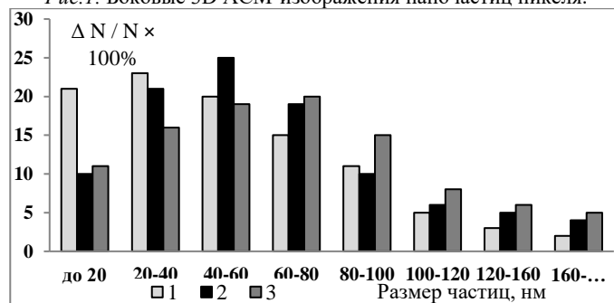
Рис. 2. Гистограммы размерных распределений наночастиц никеля. 10 8 Вт/см 2 (1), 2×10 8 Вт/см 2 (2) и 5×10 8 Вт/см 2 (3)
