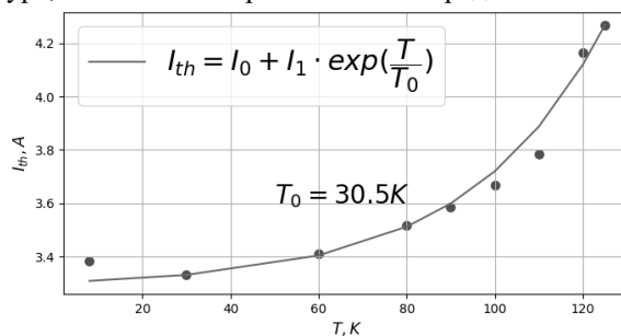
Рис. 1. Температурная зависимость порогового тока
