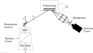
Рис. 2. Схема экспериментальной установки
