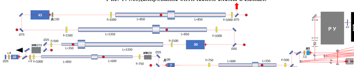
Рис. 2. Схема расположения оптических элементов и трассировки лучей.
