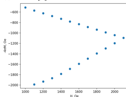
Рис. 1. Рассчитанный участок петли перемагничивания сверхпроводника YBa_2Cu_3O_{7-x}
