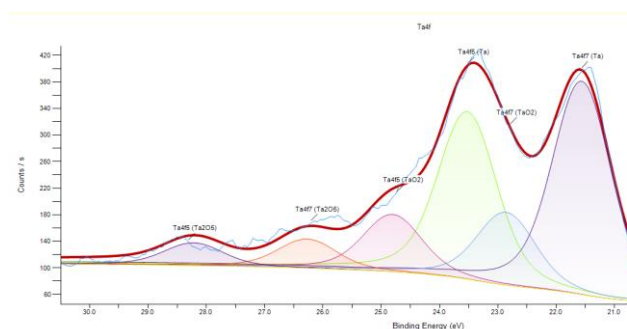
Рис. 2. РФЭС спектр нанокластеров Ta/TaO 2 /Ta 2 O 5
