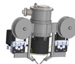
Рис. 2. Конструкция ЭЛП для двухпроволочной наплавки
