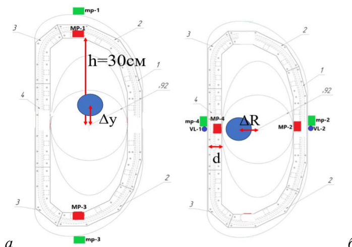
Рис. 1. Расположение электромагнитных диагностик для определения: а) вертикального смещения плазменного шнура б) горизонтального смещения плазменного шнура
