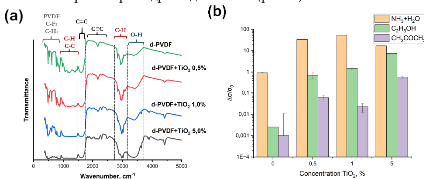
Рис. 1. ИК спектр (а) и относительное изменение проводимости при различной концентрации TiO 2 (b).
