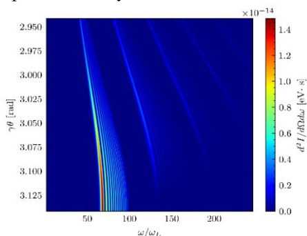
Рис. 1. Спектрально-угловое распределение рассеянного фотона с r = 2, a_0 = 1 ,
