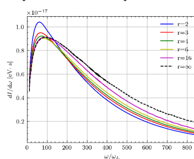
Рис. 3. Спектры рассеянного фотона, усредненные по 50 точкам с a_0 = 5, \gamma = 5, \Delta\phi = 10 и r = 2, 3, 4, 6, \infty , где \infty соответствует случаю прямоугольной огибающей
