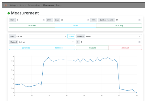
Рис. 2. Страница Web-приложения
