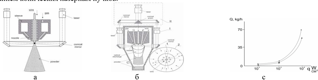
Рис. 1 Схема лазерной газовой атомизации (а); схема получения нанопорошков (б); производительность процесса: * - испарение восьми 1 mm проволок; ♠-лазерная атомизация 2 мм проволоки (с).
