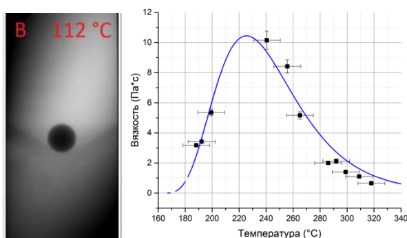
Рис.1. Слева - радиографическое изображение капсулы, заполненной расплавом серы с шариком. Справа – рассчитанное по результатам измерений значение вязкости серы (черные точки) в сравнении с теоретическими расчетами (синяя кривая)
