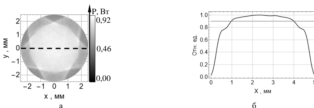
Рис.1. Пространственное распределение мощности поглощенного излучения накачки а) по поперечному сечению; б) по горизонтальному разрезу поперечного сечения активного элемента
