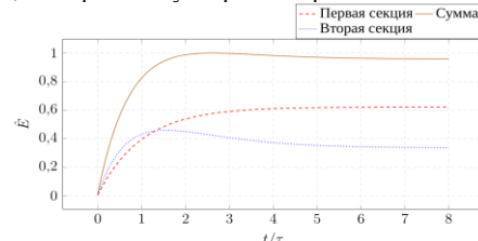
Рис. 4. Переходный режим энергии пучка в режиме низкой и высокой энергии
