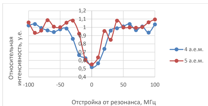
Рис. 2. Спектр флуоресценции облака ионов в зависимости от частоты часового лазера.
