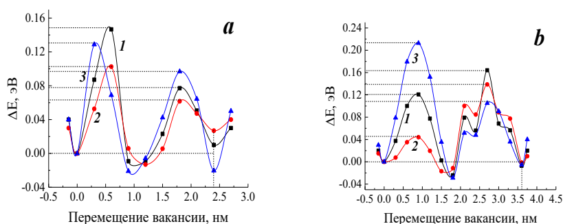
Рис. 1. Профили потенциального рельефа кристалла \text{LaF}_3 при миграции вакансии из позиции F_1 в позицию F_2 (а) и из позиции F_2 в позицию F_2 , расположенного ближе к поверхности. Кривая 1 соответствует идеальной решетке, кривые 2 и 3 – растянутой и сжатой.
