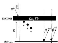
Рис. 1. Схема фотодиода
