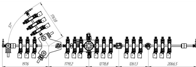
Рис. 1. Схема тракта LEBT
