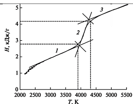
Рис. 2. Энтальпия H этого же карбида [2].
