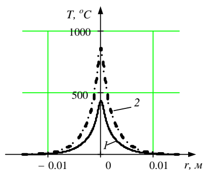
Рис. 1 Расчетные варианты распределения температуры
