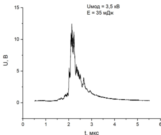
Рис. 1. Оциллограмма модулированного лазерного импульса с длительностью \sim 0,3 мкс по полувысоте
