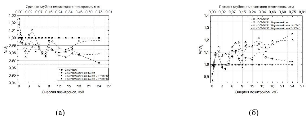
Рис. 1. Зависимости S/S_0 (а) и W/W_0 (б) позитронов переменной энергии в НМС Zr/Nb 50 нм после облучения ионами гелия и последующего отжига при различной температуре
