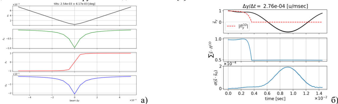
Рис. 1. а) Спин-флиппинг при прохождении резонансной энергии в QFS-структуре;
