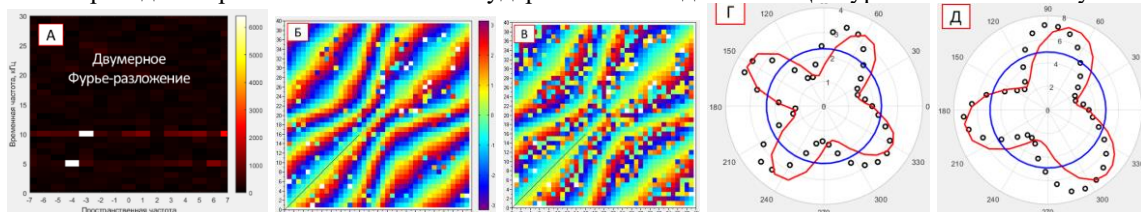
Рис. 1 А – Матрица двумерного Фурье-разложения композиции мод с полоидальными модовыми числами m=4 и m=3
