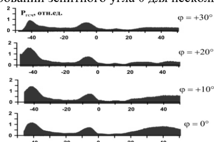
Рис. 1. Зависимость P_{\text{Гсч}} от зенитного угла \theta для различных значений азимутального угла \varphi
