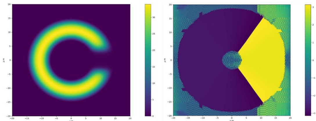
Рис. 1. Пространственный профиль плотности(слева) и фазы(справа) основном состоянии (единицы измерения \frac{1}{\mu\text{m}^2} ).
