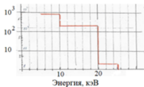
Рис. 2. Спектр РИ
